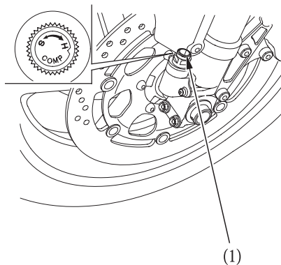
(1) Регулятор демпфирующего усилия
