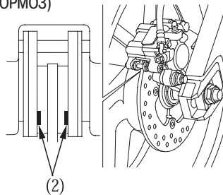
(2) Вырезы
